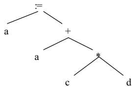
Figura 1.1. Árvore de sintaxe da expressão a := b + c * d .
