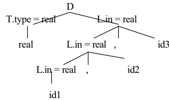
Figura 4.2. Árvore de derivação com o atributo herdado in em cada nodo L .
