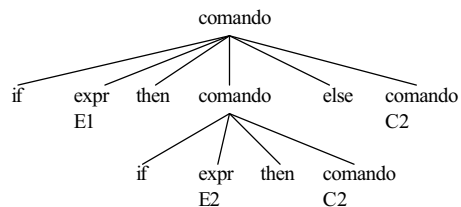
Figura 3.2. Árvores de derivação para gramática ambígua.
