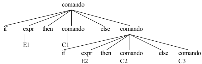
Figura 3.1. Árvore de derivação para o comando condicional.
